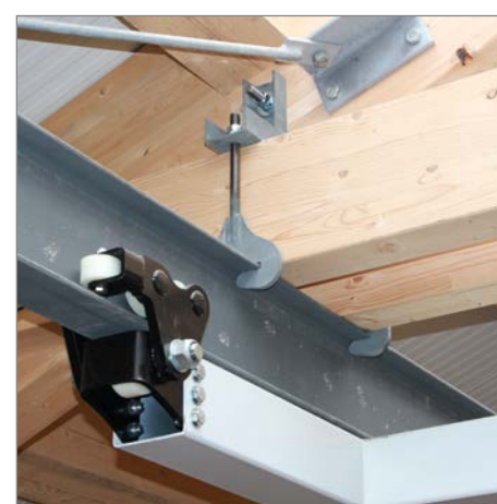
verschiedenste Schienenkonsolen
