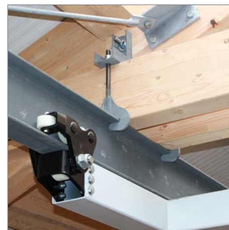
verschiedenste Schienenkonsolen
