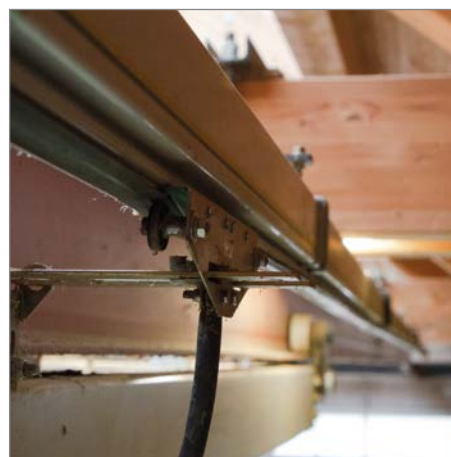
Schleifleitungskanal
